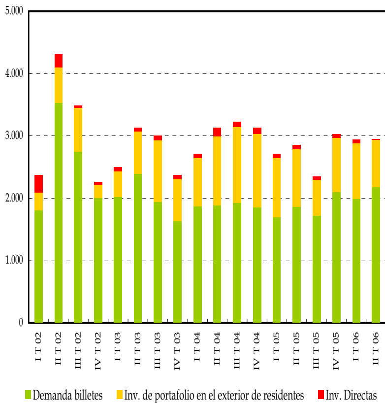
Demanda bruta
