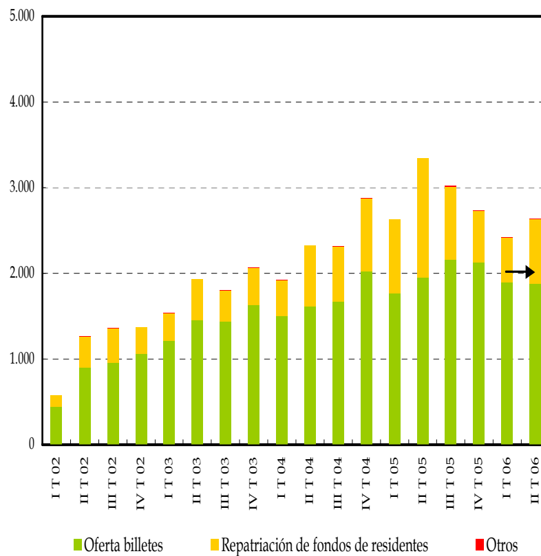
Oferta bruta
